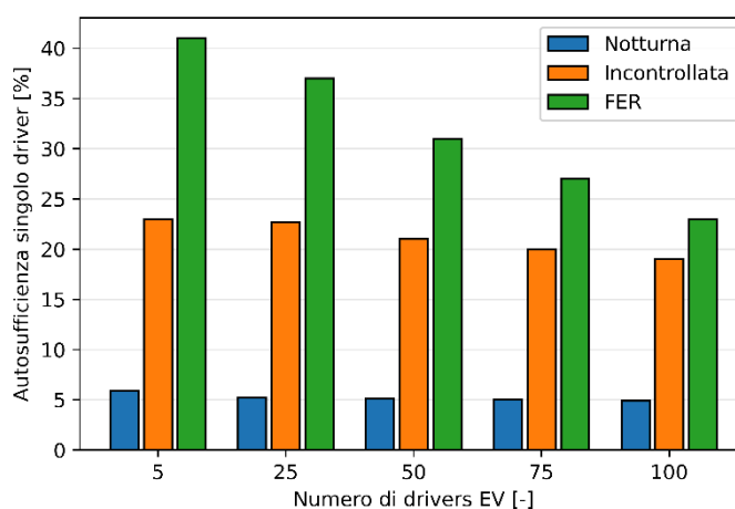
Figura 14: Autosufficienza singolo driver CER per le tre strategie di ricarica.
